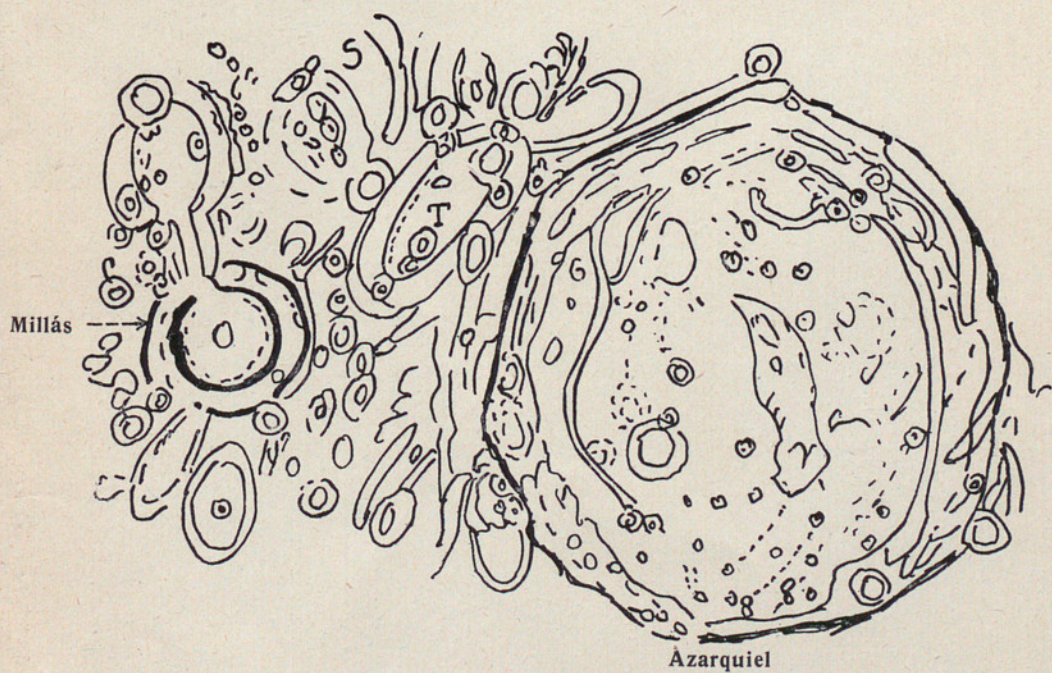
Cráter MILLÁS que aparece en la tercera edición del Mapa Lunar de H. P. Wilkins Dibujo del mapa de H. P. Wilkins, reducido a 100 pulgadas. (Fotografía del Observatorio Lick)
