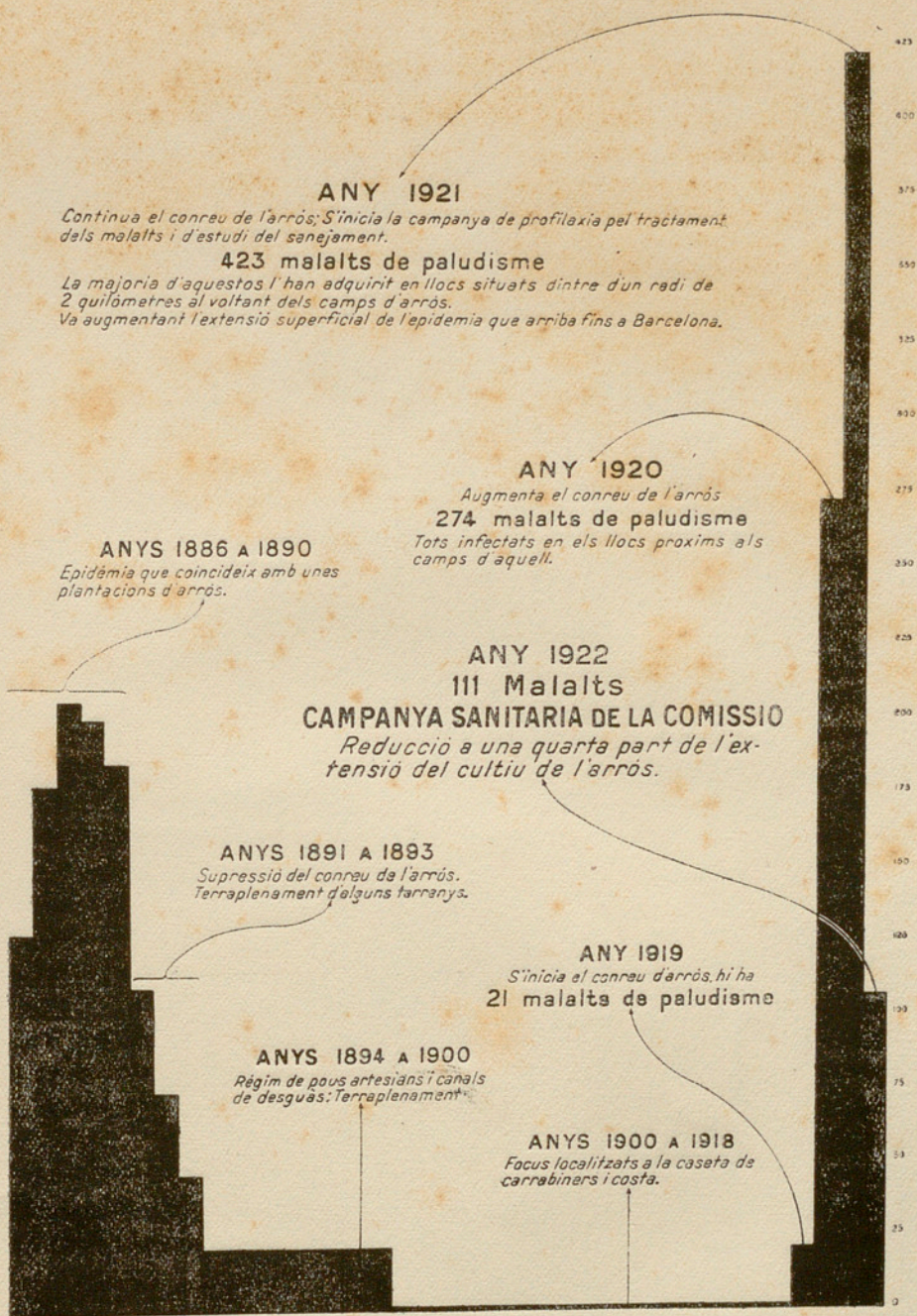
Gràfic de la morbiditat palúdica en el Prat de Llobregat des de 1886 a 1922
