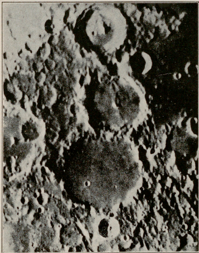
FIG. 2. a — REGIÓ LLUNAR PROPERA AL CIRC DE TOLEMAUS Fotografia obtinguda a l'Observatori de Mount-Wilson amb un telescopi de 33 cm.
