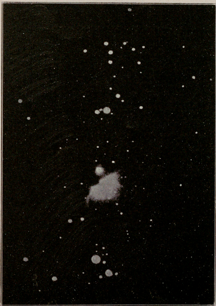
FIG. 5. a — LA GRAN NEBULOSA D'ORIÓ
