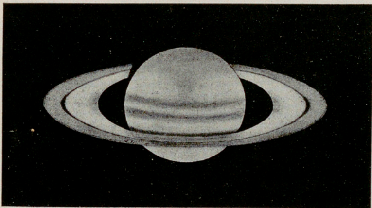
FIG. 4. a — EL PLANETA SATURN
