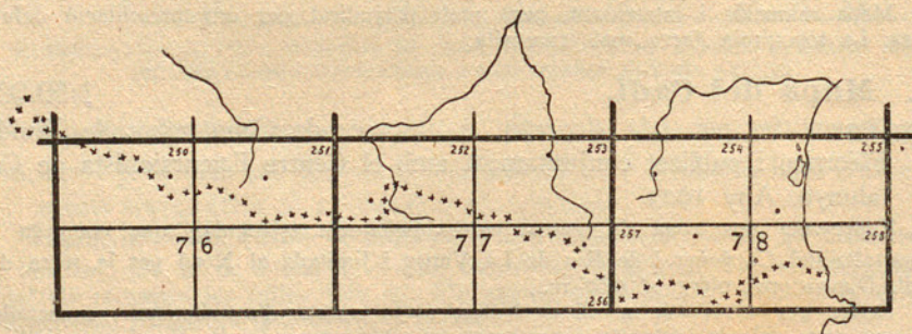
4. Fulles corresponents a Catalunya i als Pirineus centrals dels mapes de França a 1/80.000 (divisió i xifres petites) i a 1/200.000 (divisió i xifres grans).
