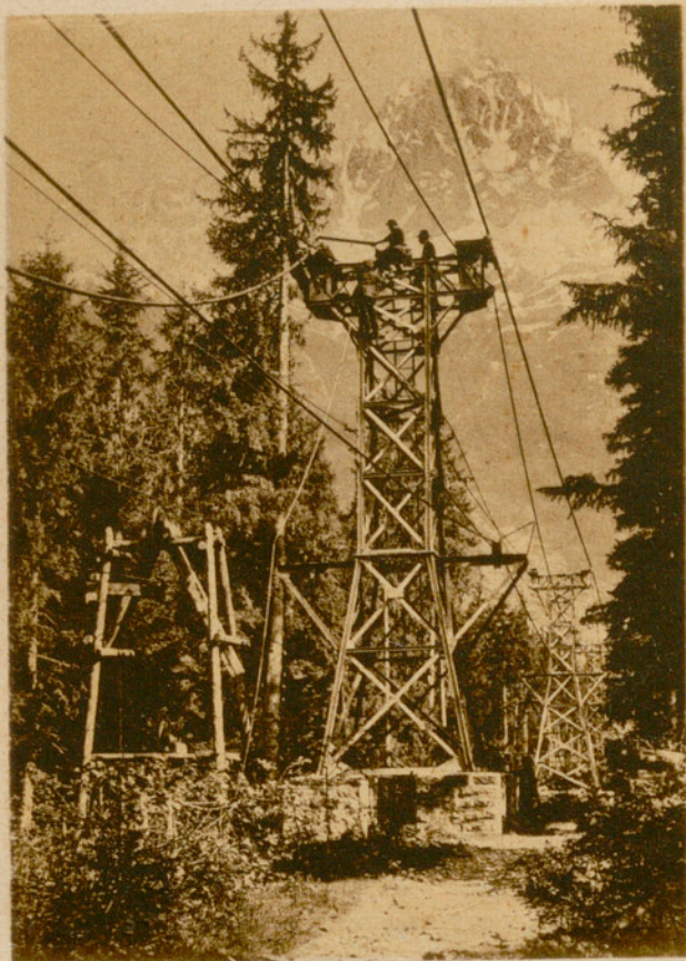
UN PYLONE PENDANT LE MONTAGE DES CABLES.
