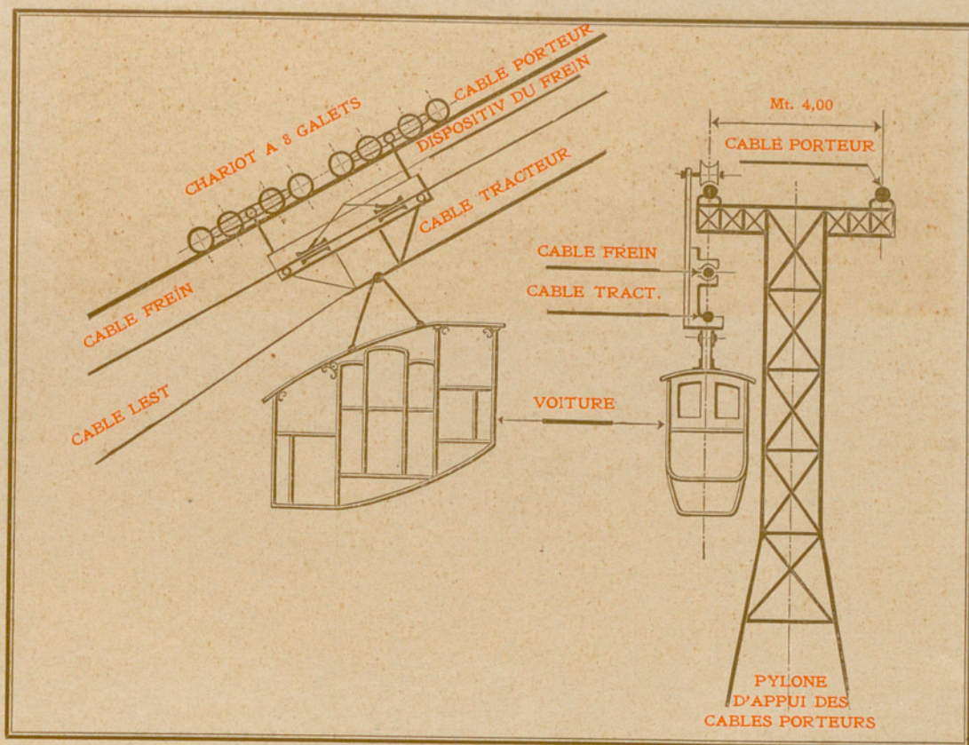
ELEVATION SCHEMATIQUE DU CHARIOT AVEC VOITURE ET PYLONE.
