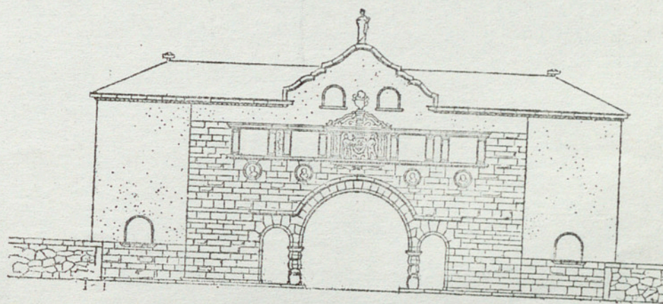
Fig. 19. — FAÇADE DU PAVILLON DU CONCIERGE (H).
