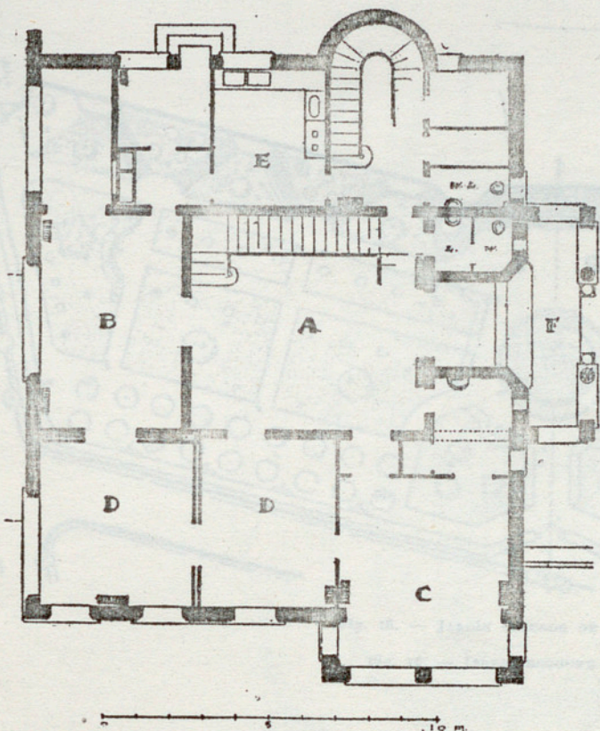
Fig. 14. — PLANTA BAJA DEL PABELLÓN DEL DIRECTOR (T). A, Hall; B, Comedor; C, Despacho; D, Salitas de recepción; E, Cocina; F, Entrada al pabellón.
