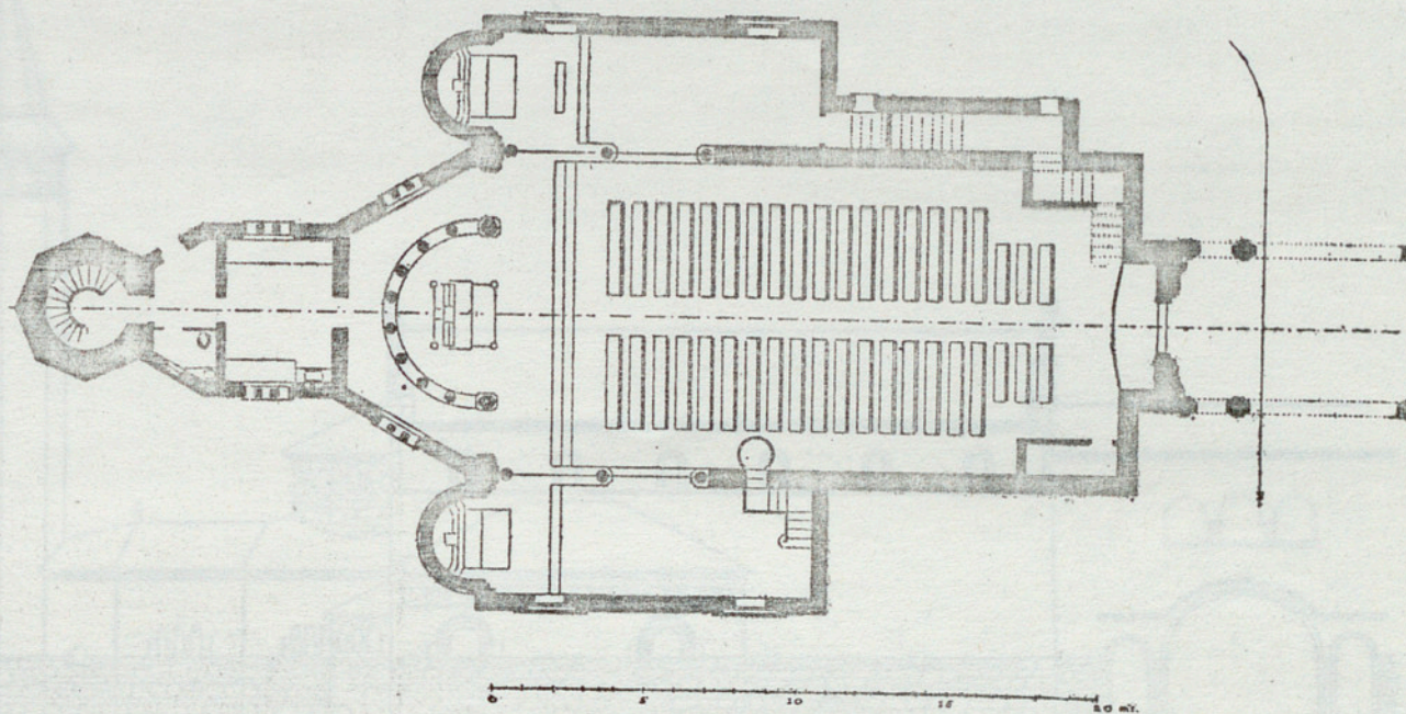
Fig. 12. — PLANTA BAJA DE LA IGLESIA (U).
