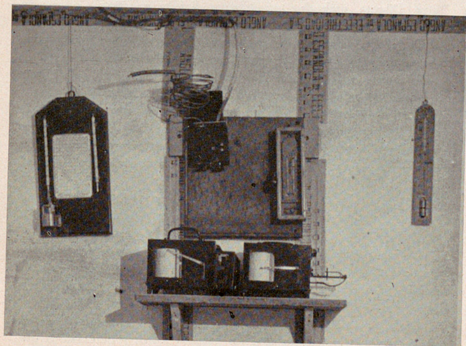
Fig. 2.—Quadre d'aparells registradors
