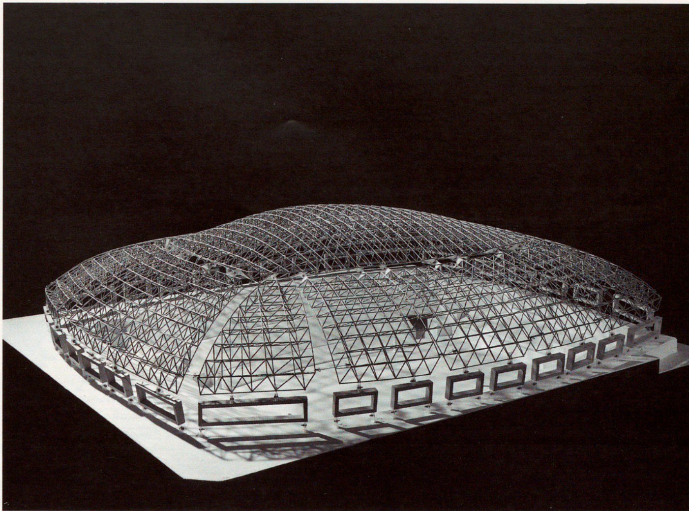
UN DELS ASPECTES MÉS INNOVADORS DEL NOU PALAU ÉS L'ESTRUCTURA QUE DÓNA SUPORT AL SOSTRE DE L'OBRA
