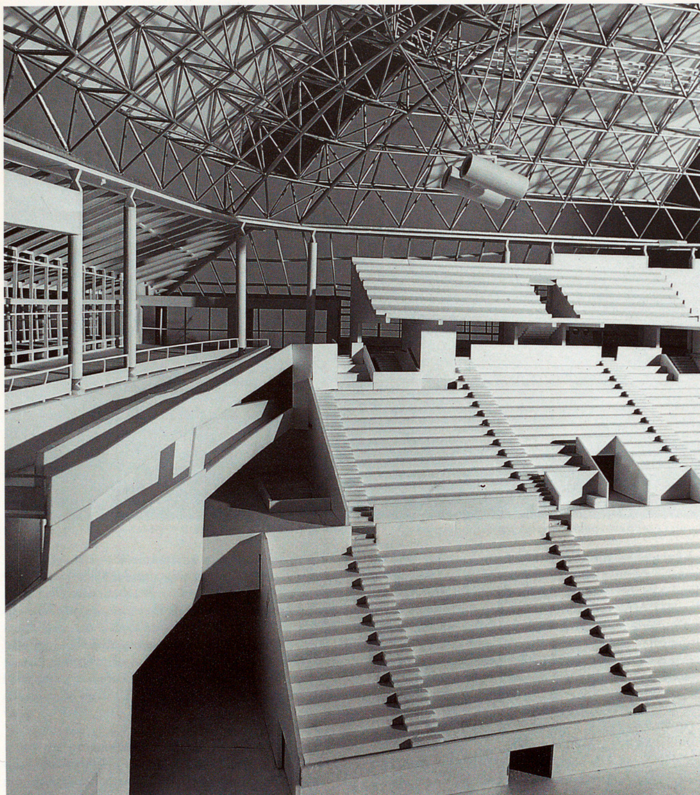
LES GRADES MÒBILS DEL PALAU, QUE PERMETRAN D'AMPLIAR L'ESPAI SEGONS LES DISCIPLINES ESPORTIVES
