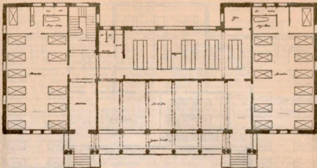
Pavelló per a epilèptics. Planta baixa
