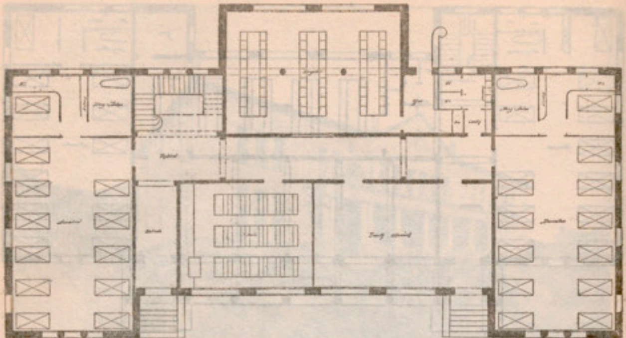
Pavelló per a tuberculosos (infants) : Planta baixa
