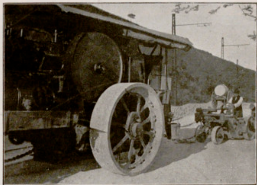
8. — Trepitjadora de 15 tones i tipus modern alemany, d'escarificadora independent de la locomòbil
