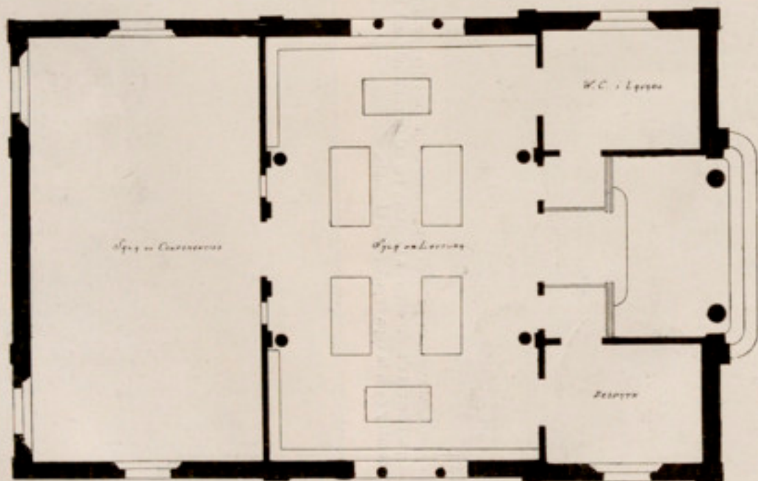
PLANTA DE L'EDIFICI
