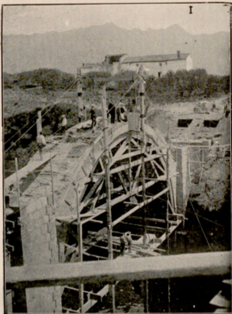
I. Col·locació de les claus de l'arc central, el pes de les quals és de 1.500 qgs., a una alçada de 25 metres, al pont d'enllaç entre els Bruchs d'Abaix i del Mig amb el de la Parròquia. — II. Arc central de 20 metres, i pila i estreb de la dreta del pont d'enllaç entre els Bruchs d'Abaix i del Mig amb el de la Parròquia. — III. Peraltament de corba i contracorba a la carretera de Monistrol a Montserrat.
