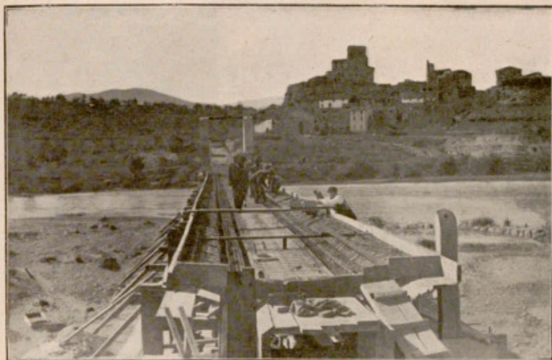
PONT DE VERNET SOBRE EL RIU SEGRE
