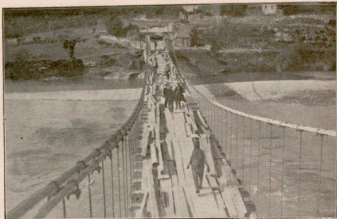
PONT DE VERNET, SOBRE EL RIU SEGRE El tram penjat, de 70'30 m. de llum, en construcció
