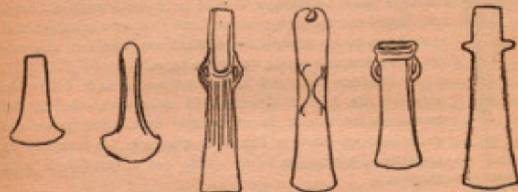
Fig. 34.—Tipologia de les destrals de bronze de la Península
