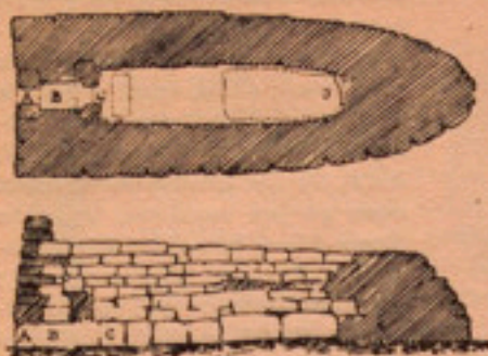
Fig. 37.—Planta i secció de la naveta dels Tudons (Clutadella)
